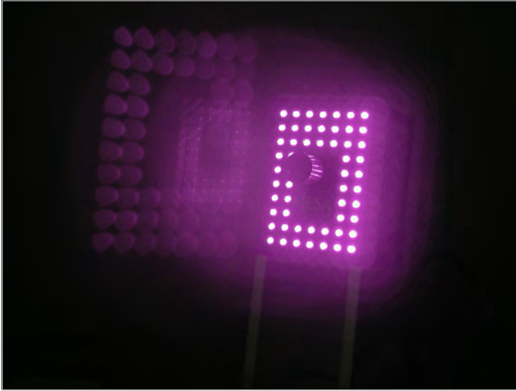
3D-Kamera in Aktion: der Sensor der Digitalkamera kann Infrarotlicht besser wahrnehmen als das menschliche Auge
